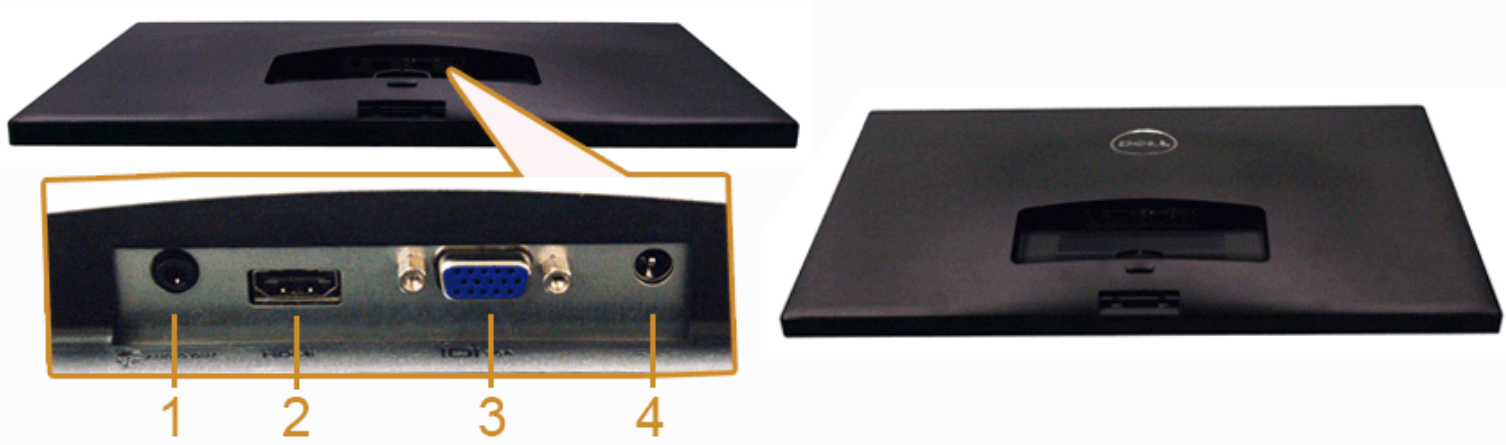
モニタスタンドなし底面図
